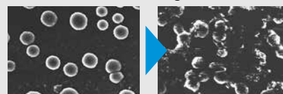
Virus voor en na bestraling
