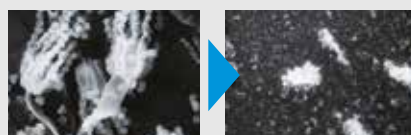
Allergeen op basis van pollen voor en na bestraling
