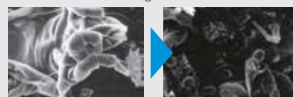
Schimmelallergeen voor en na bestraling
